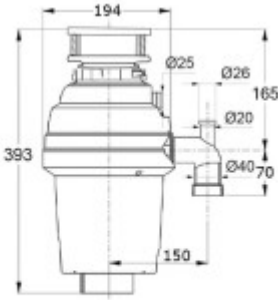
EcoMaster EVO3 LCD
